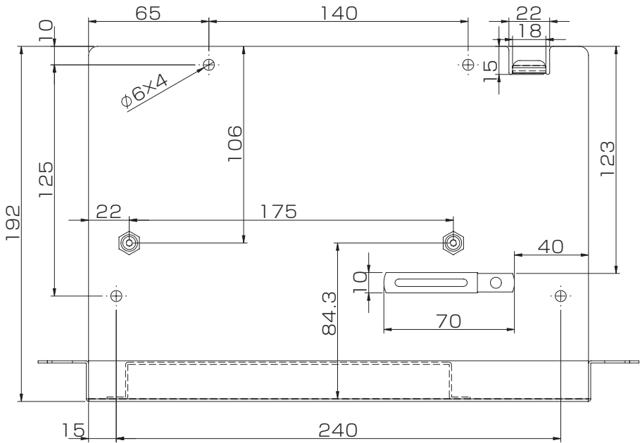
正面図
