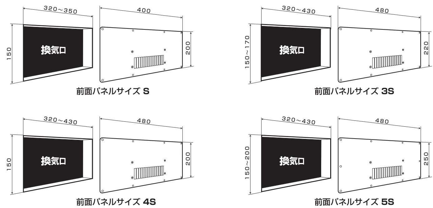
前面パネルサイズ別対応換気口寸法 [単位：mm]
