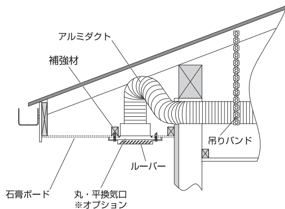
軒天ヘダクトが通るスペースがある場合の取付
