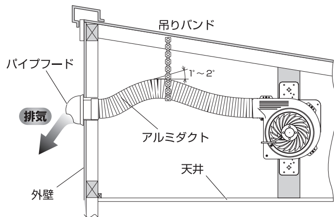
パイプフードタイプ
