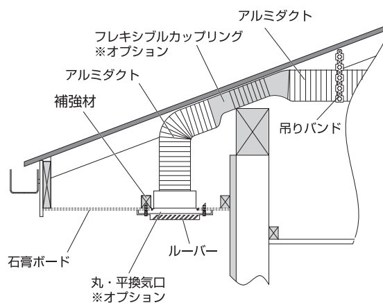
フレキシブルカップリングを利用しての取付
